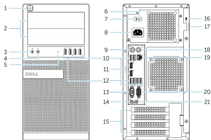
図 1. ミニタワーの正面図と背面図
